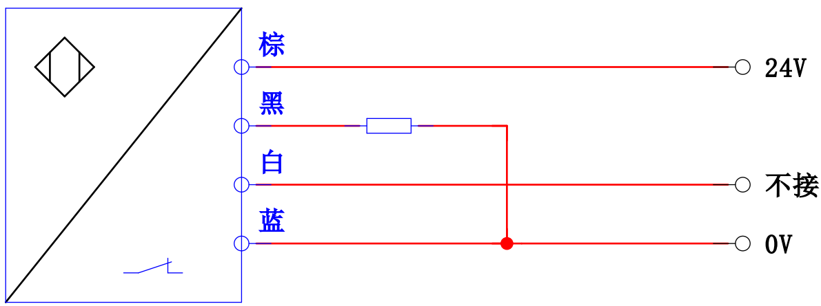
PNP-NC接线方式
