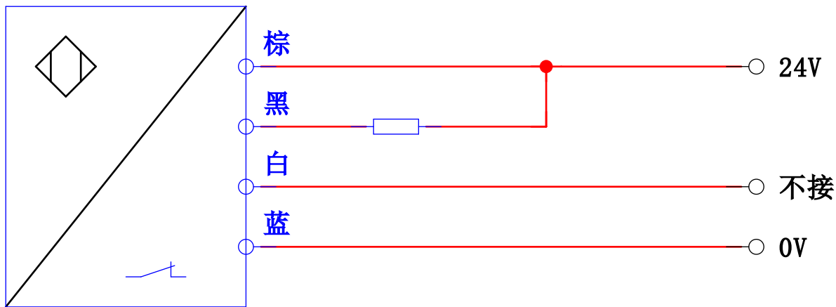
NPN-NC接线方式
