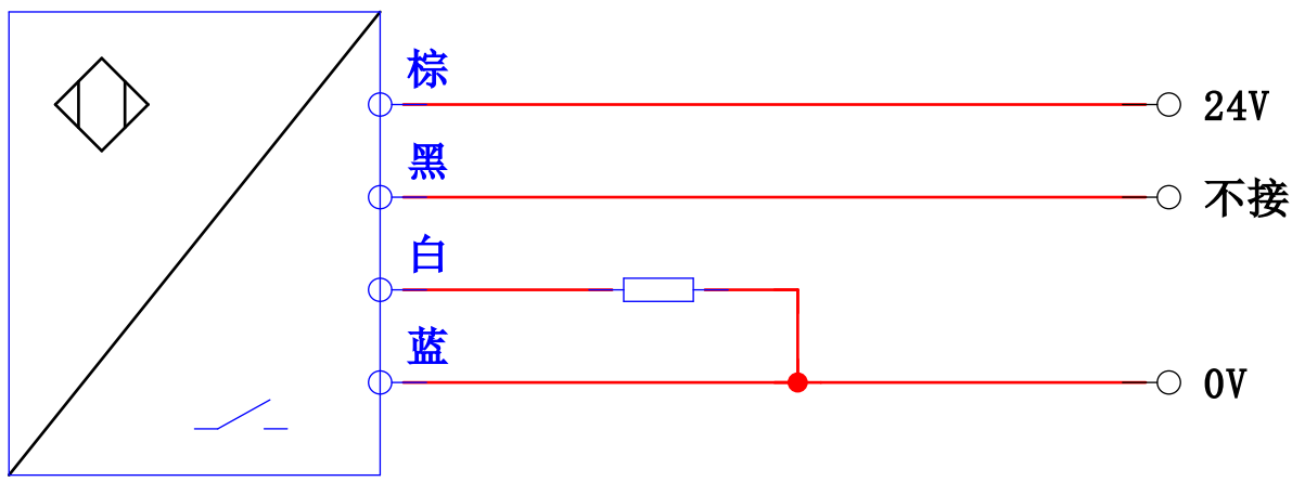
PNP-NO接线方式
