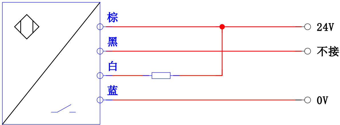
NPN-NO接线方式
